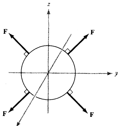
Figura 7.2.3 Campo vectorial \mathbf{F} normal a un círculo en el plano yz .
